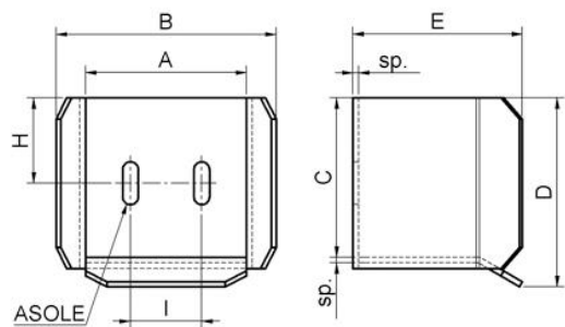
Suport de suspendare – Art. 397 M
