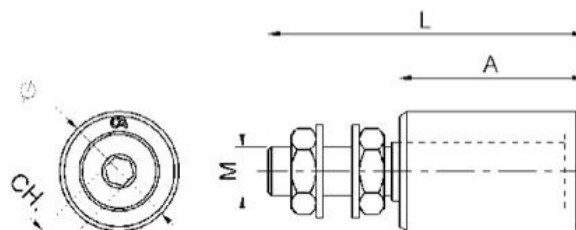
Roală superioară – Art. 450 fi 30 x 40 M 14
