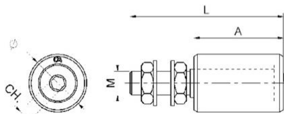
Rolă superioară – Art. 450 fi 30 x 40 M 14
