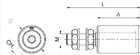
Rolă superioară – Art. 450 fi 30 x 40 M 14
