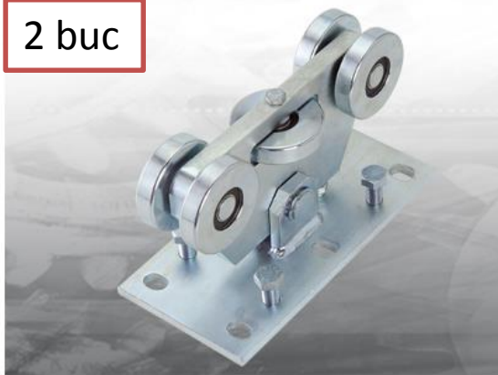
Grup de rulmenți – Art. 395 M
